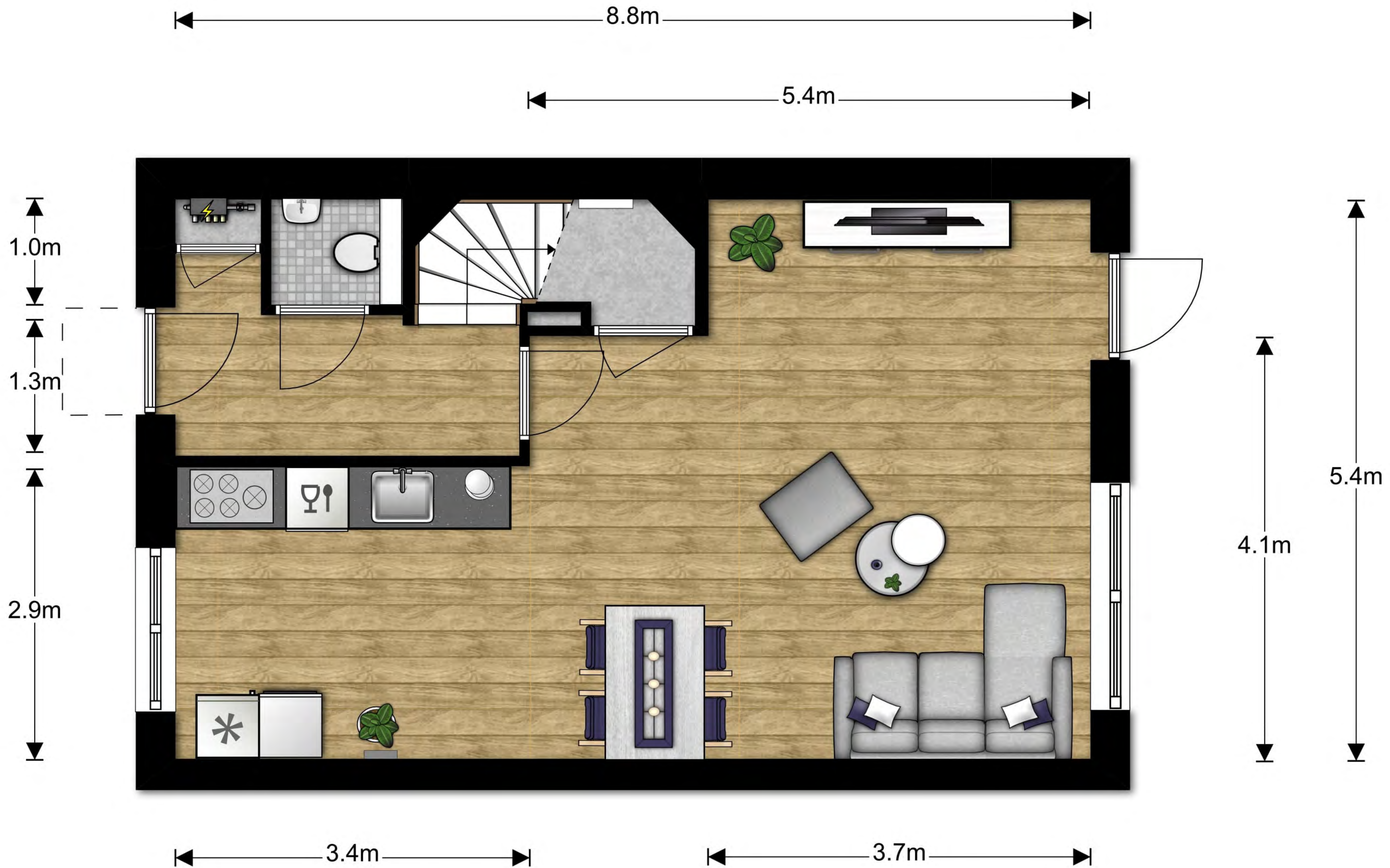
Begane grond, Oisterwijk, Schaverij 51
